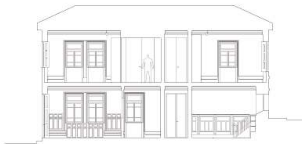
CORTE LONGITUDINAL
