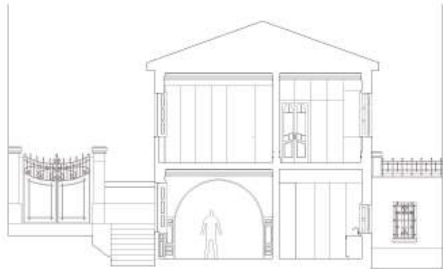
CORTE TRANSVERSAL
